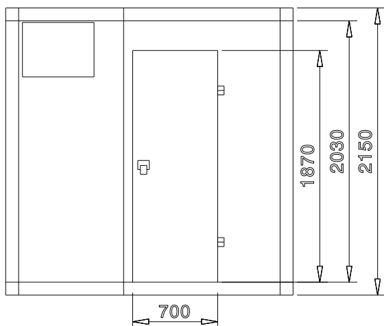
Przód
